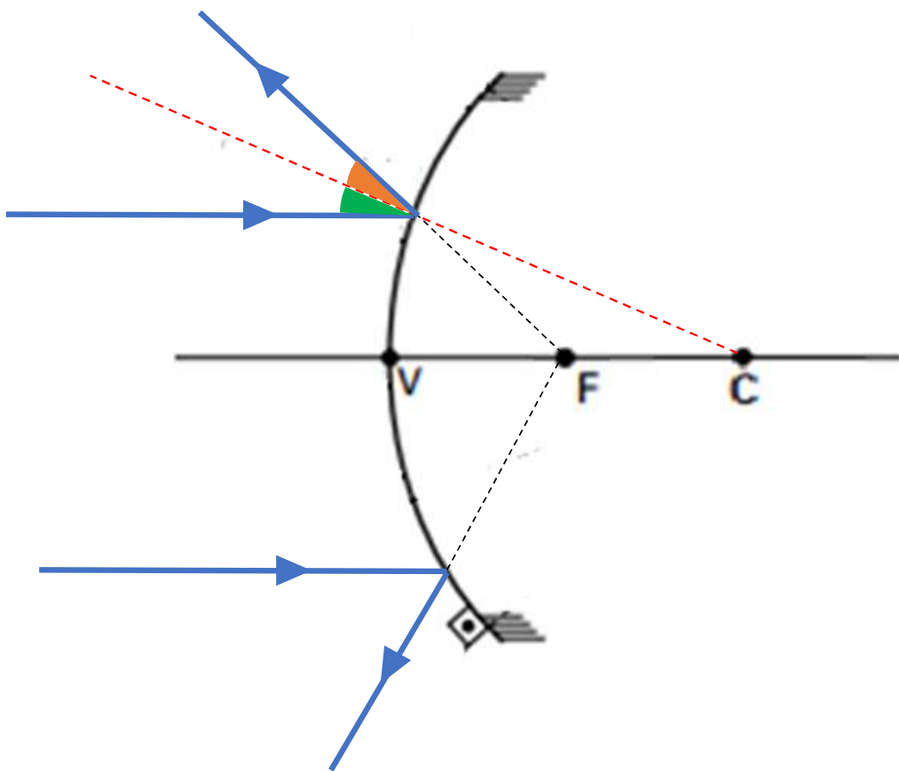
ESPELHO CONVEXO
